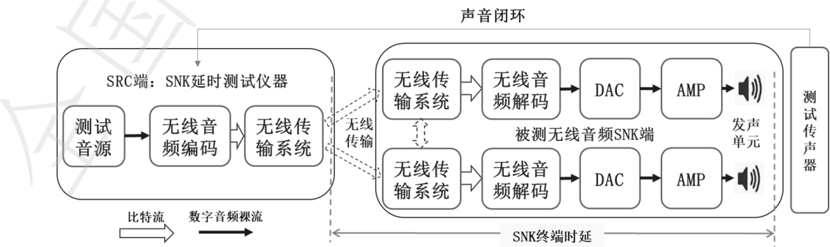
图6 SNK时延测试组网及时序示意图
