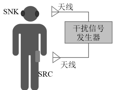
图3 贴身携带场景测试环境示意图
