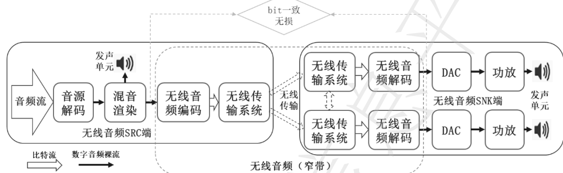
图1a 无损无线音频系统音频播放流程图（窄带）
