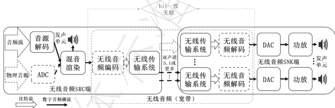
图1b 无损无线音频系统音频播放流程图（宽带）
