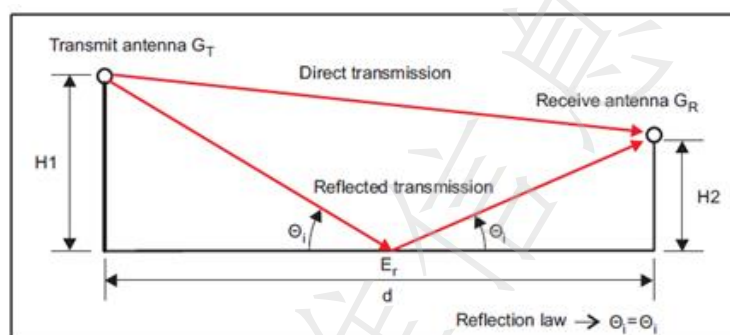
图A1 地面反射模型示意图
